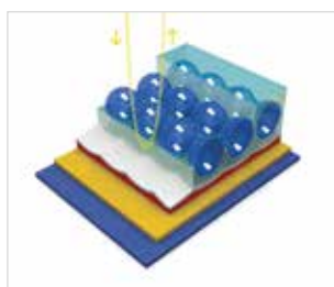
Funkční diagram retroreflexní folie Typ 1 = třída R1
