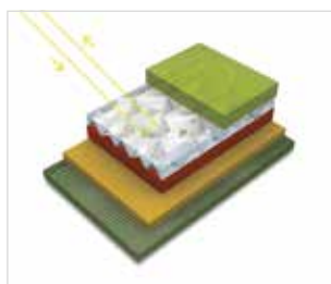
Funkční diagram retroreflexní folie Typ 2 = třída R2
